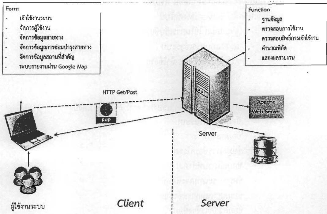
ภาพแสดงสถาปัตยกรรมของระบบข้อมูลสายทางจังหวัดลพบุรี
